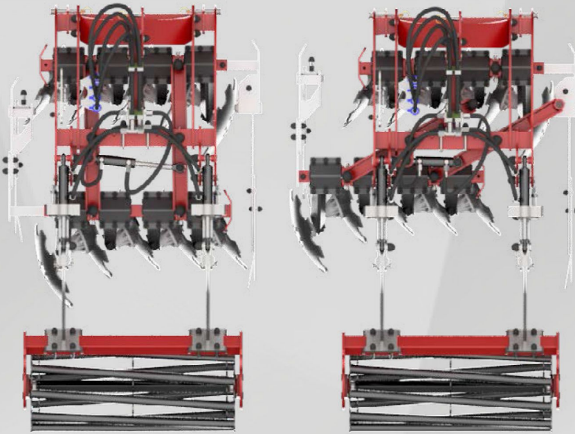
Hidraulikus munkaszélesség állítás
