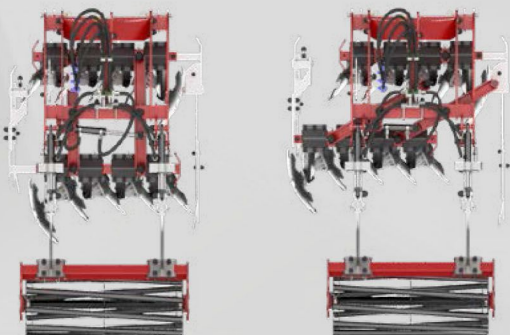
Hidraulikus munkaszélesség állítás
