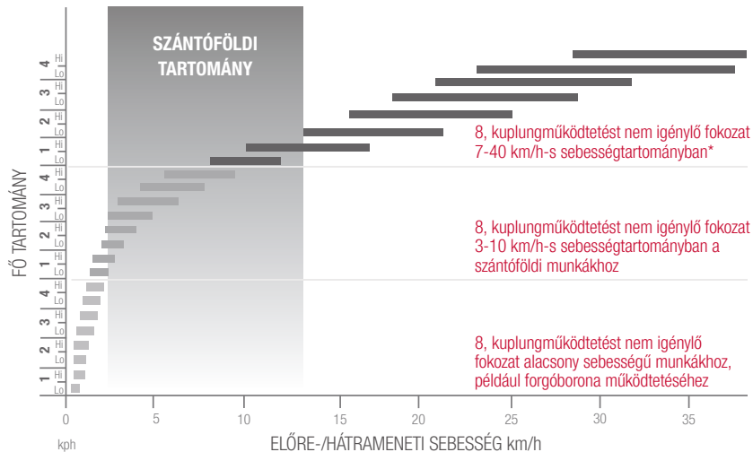
24x12 SPEEDSHIFT FOKOZATKIOSZTÁSI DIAGRAM
